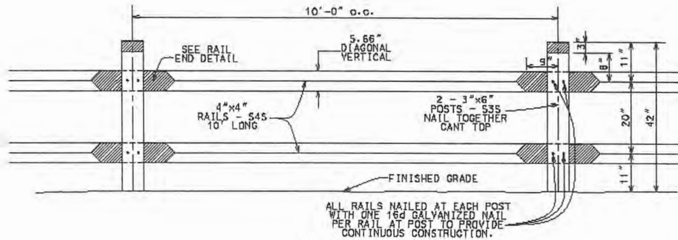
ELEVATION SCALE: 1" = 20'
